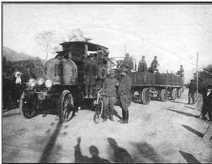
Locotenentul Konrad Twrdy însoțind un tren benzino electric încărcat cu materiale, spre șantierul căii ferate de pe Tihuța foto din colecția Kurt Misar și Martina Misar-Tummeltshammer
