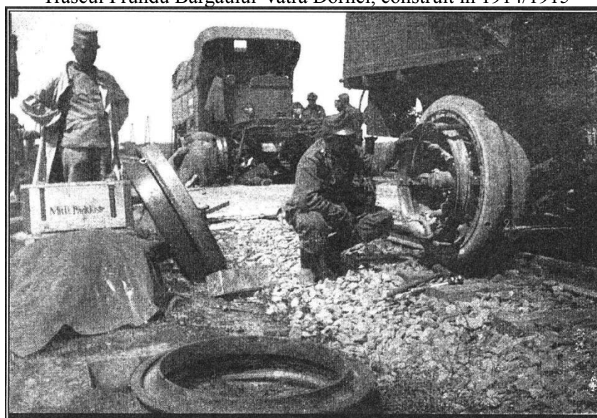
Montarea jantelor speciale pentru deplasarea pe calea ferată la un auto-tren - arhive Austria
