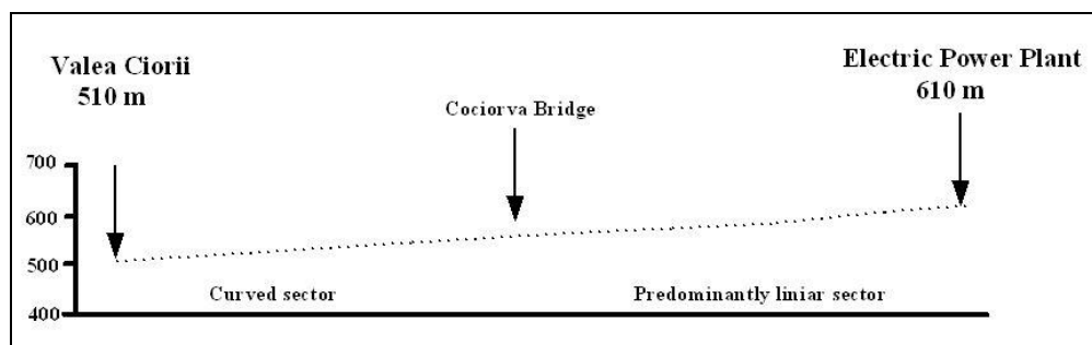
Fig.3-Profilul longitudinal al sectorului de râu folosit pentru rafting controlat
