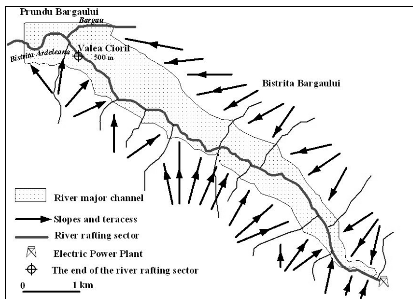
Fig.4-Schiță geomorfologică a sectorului de râu folosit pentru rafting controlat
