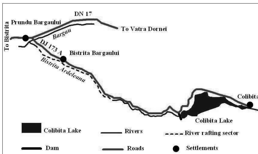
Fig.2-Sistemul hidrografic Lacul Colibița-Râul Bistrița Ardeleană
